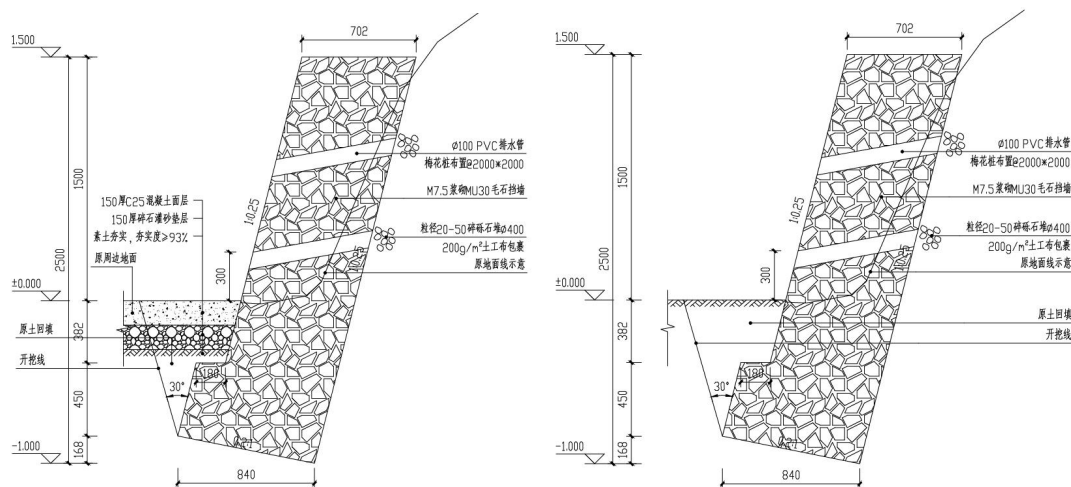
图 3-51 1.5m 高挡墙大样图
