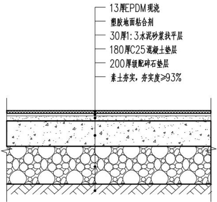
图 3-83 橡胶地面做法
