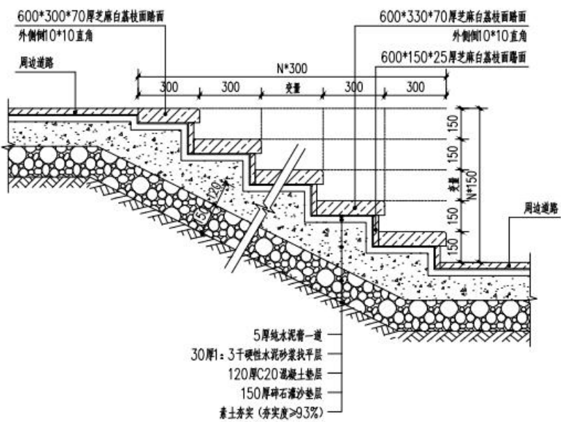
图 3-23 台阶做法大样图
