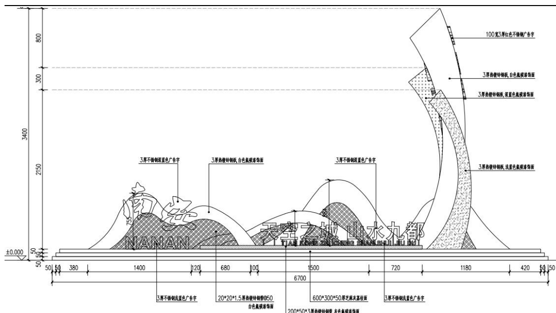
图 3-38 镇标做法
