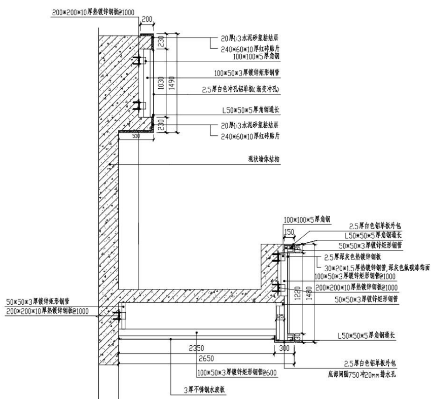
图 3-6 移民文化展示中心 2-2 断面图
