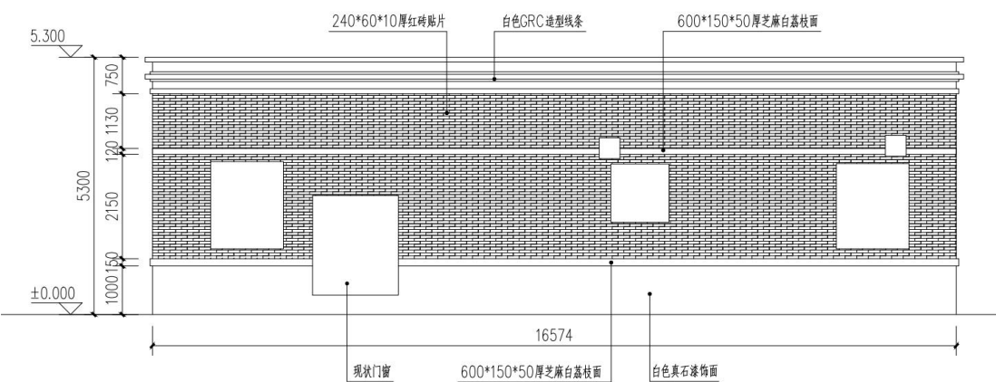
图 3-14 水泵房一立面图 B
