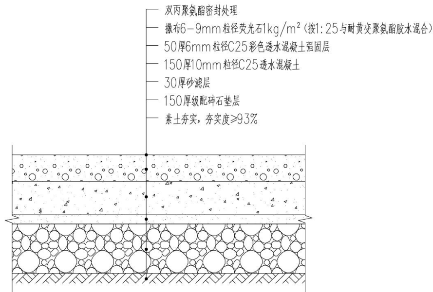
图 3-25 透水混凝土道路做法
