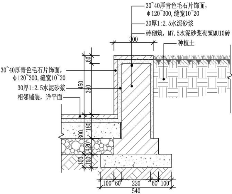
图 3-93 花池做法
