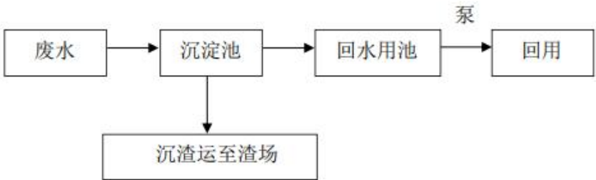
含泥沙施工废水处理工艺流程图 1
