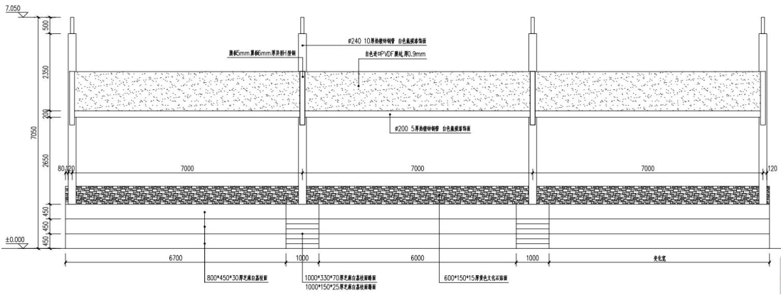
图 3-19 移民文化广场看台立面图
