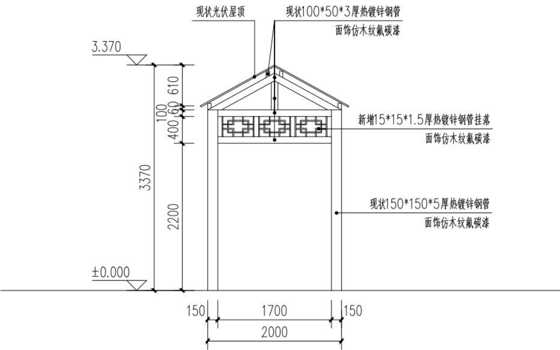
图 3-41 休闲长廊提升做法
