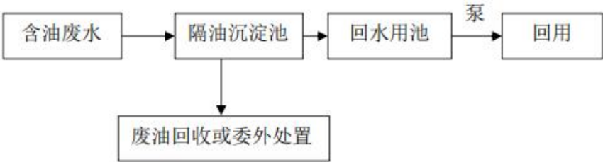
含泥沙施工废水处理工艺流程图 2
