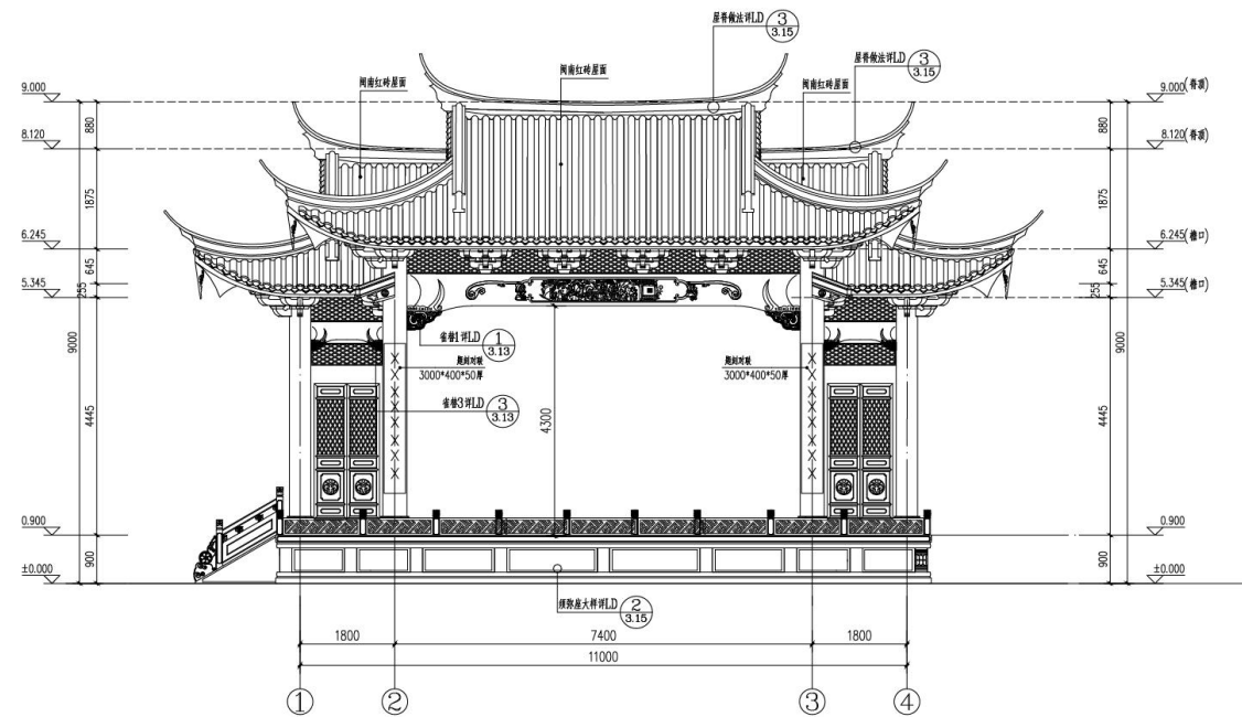
图 3-9 戏台正立面图
