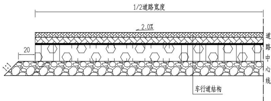
图 3-70 路面改造结构形式三（适用于土路新建路面结构段）
