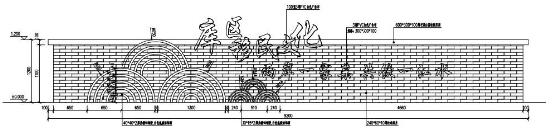
图 3-76 库区移民文化展示墙立面做法
