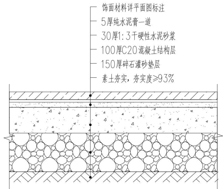
图 3-26 石材铺装地面做法
