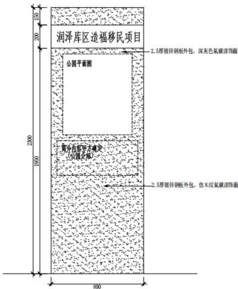
图 3-54 展示牌立面做法
