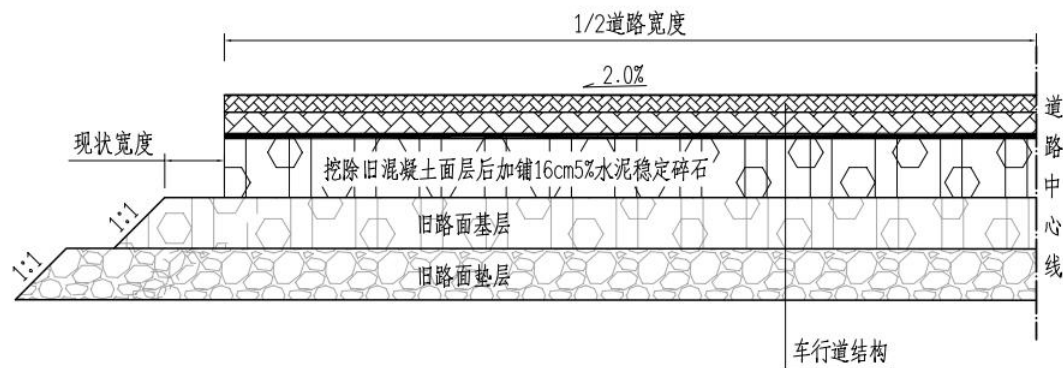
图 3-69 路面改造结构形式二（适用于旧路面挖除后加铺沥青段）
