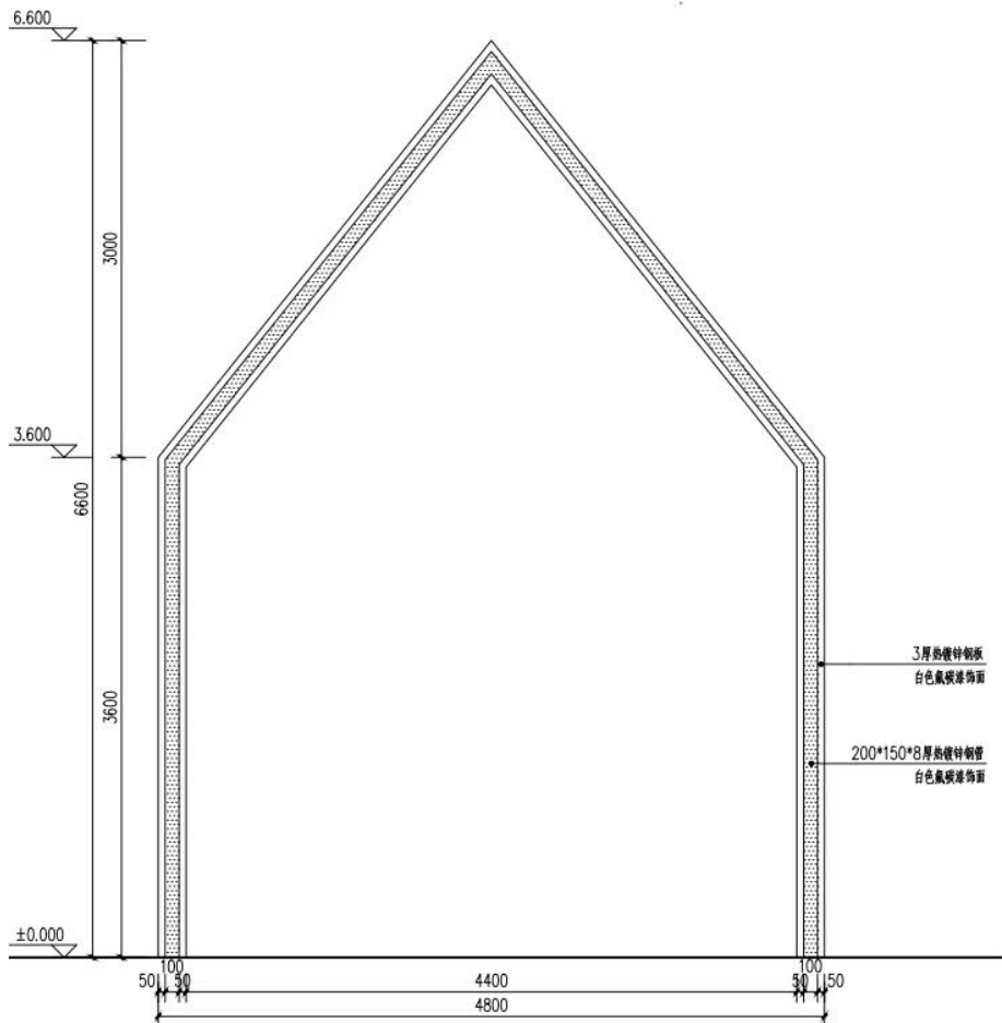
图 3-35 白色塔形廊架做法
