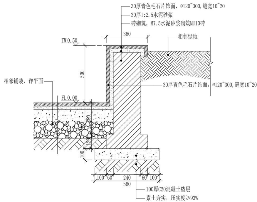
图 3-90 挡墙做法
