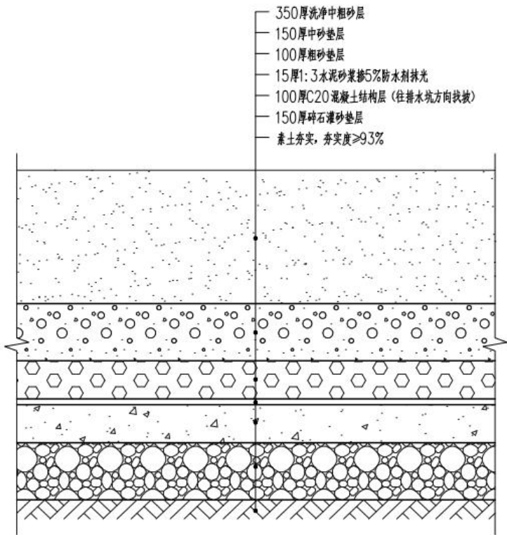
图 3-84 沙坑地面做法
