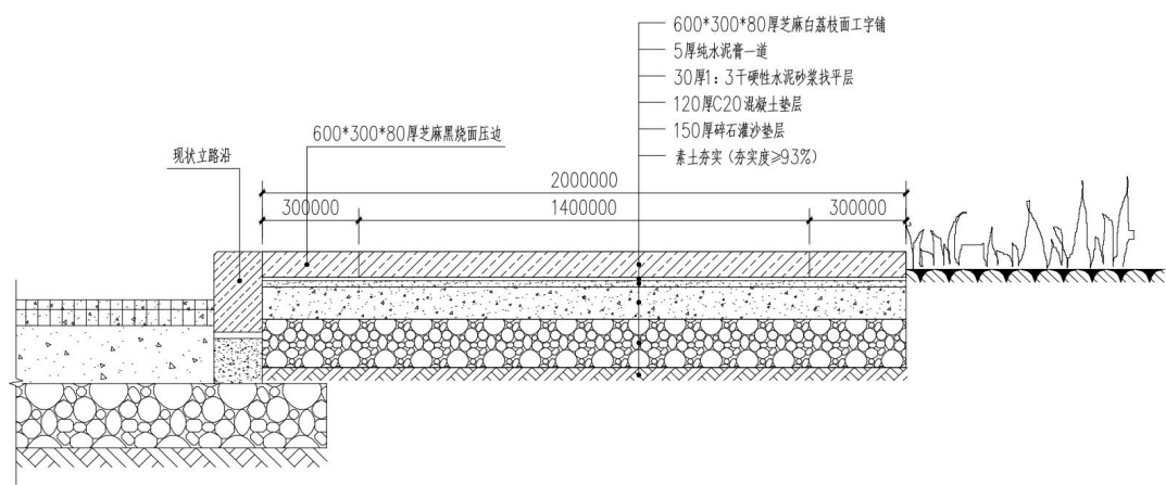
图 3-27 人行道做法
