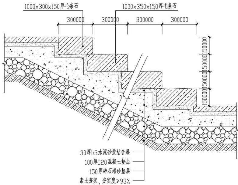
图 3-47 条石台阶做法
