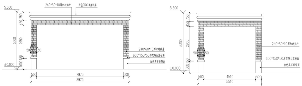
图 3-16 水泵房二正、侧立面图
