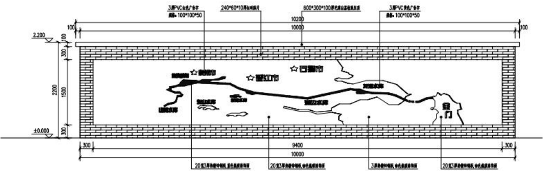
图 3-77 金門供水文化展示墙做法
