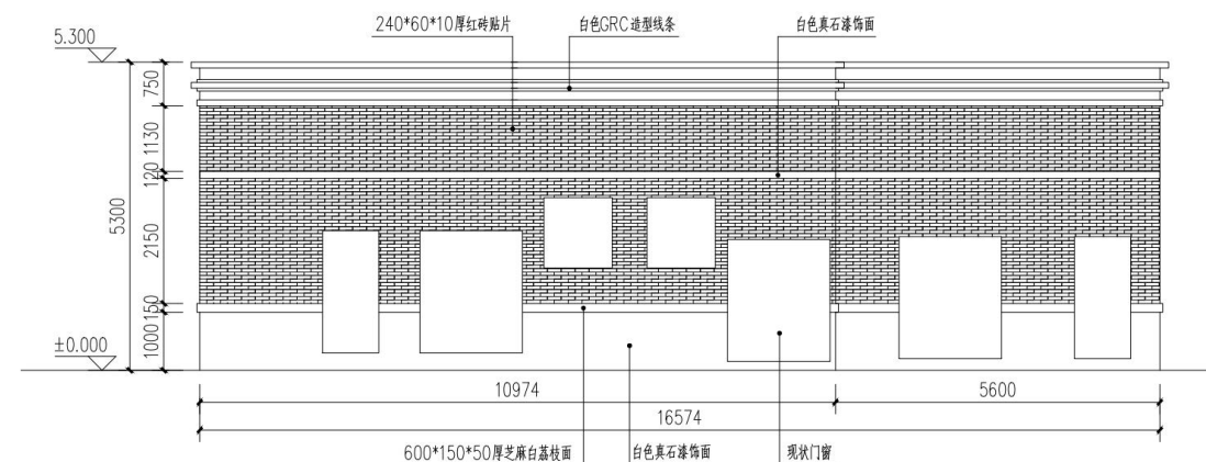
图 3-13 水泵房一立面图 A
