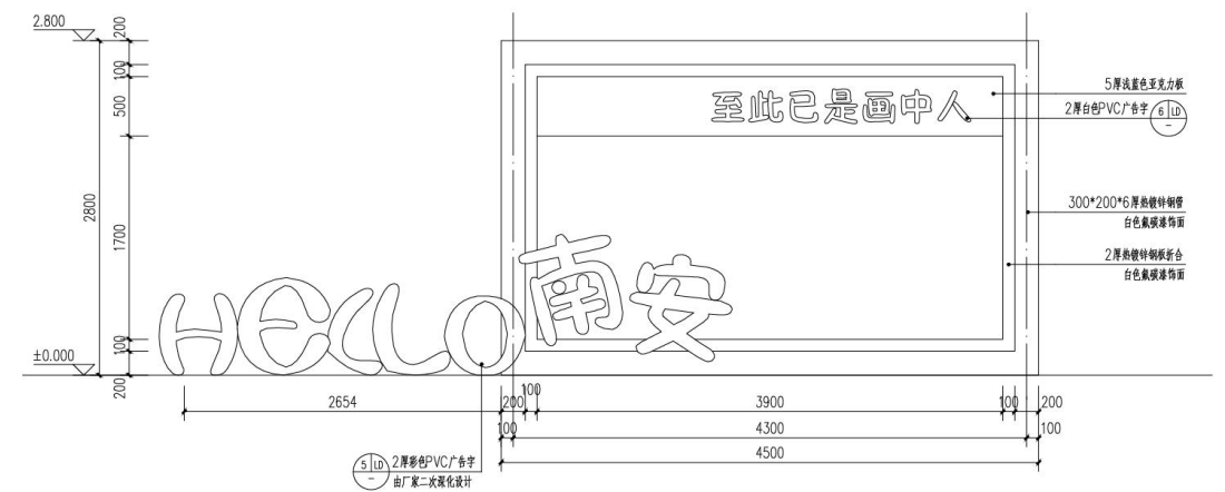
图 3-32 打卡画框做法
