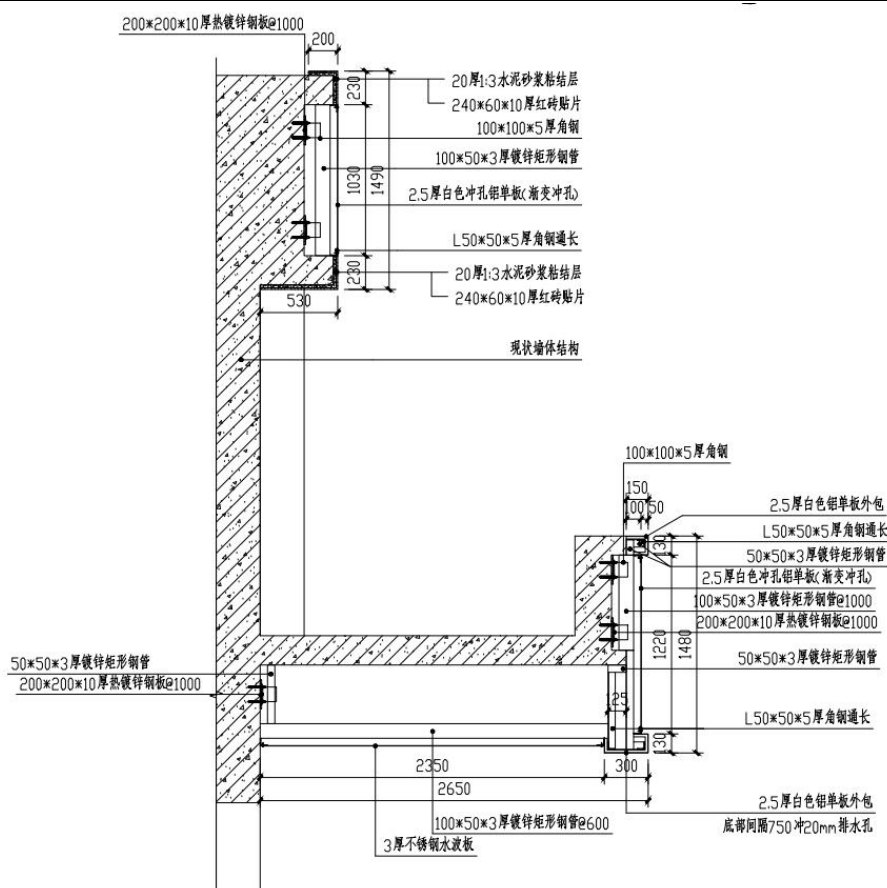
图 3-5 移民文化展示中心 1-1 断面图
