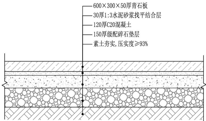
图 3-87 步道提升做法
