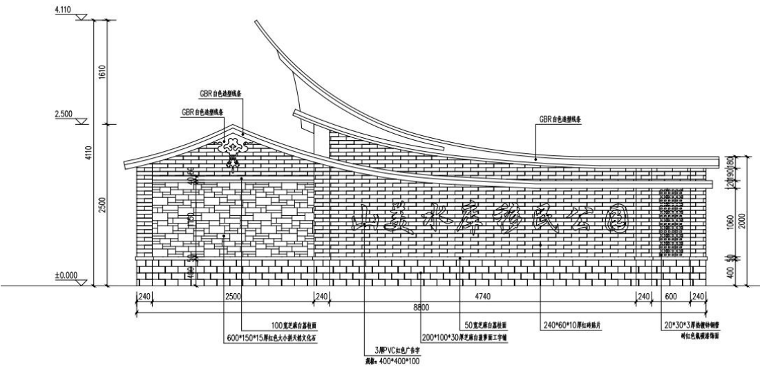
图 3-73 入口案名景墙做法
