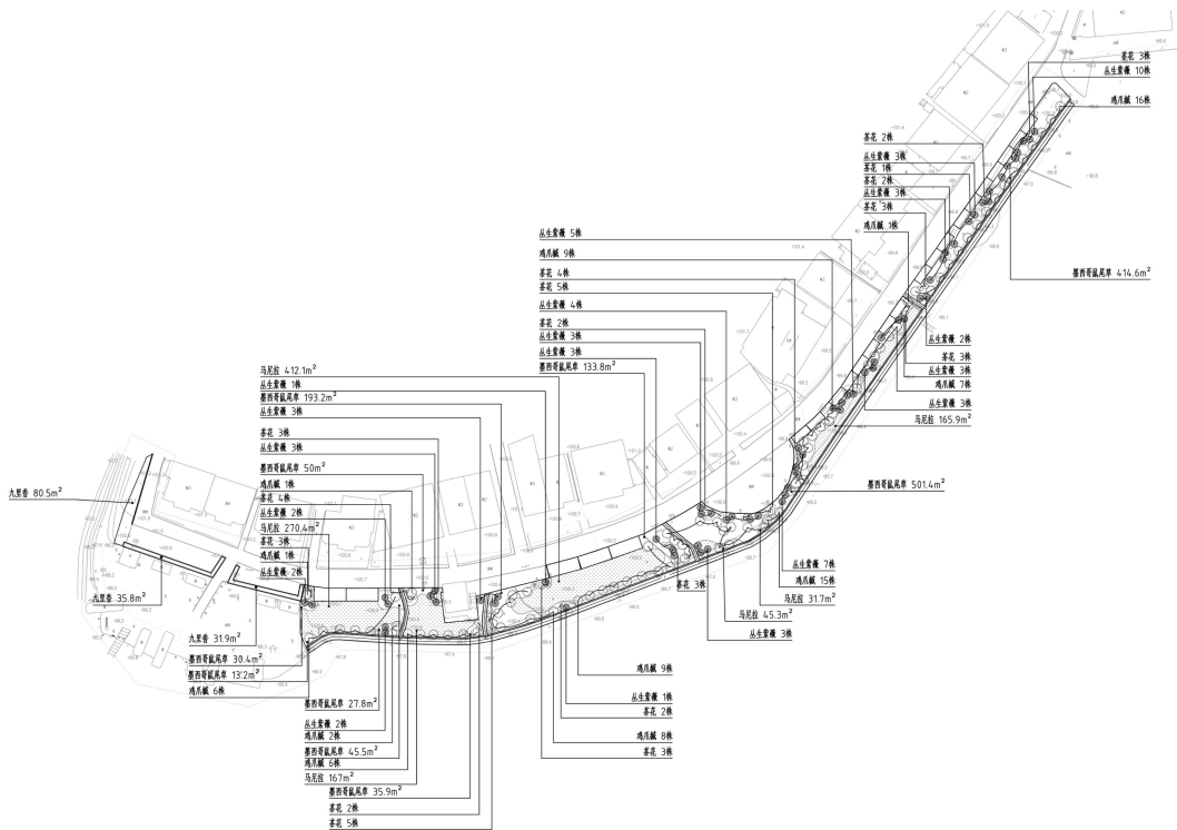
图 3-98 绿化布置图
