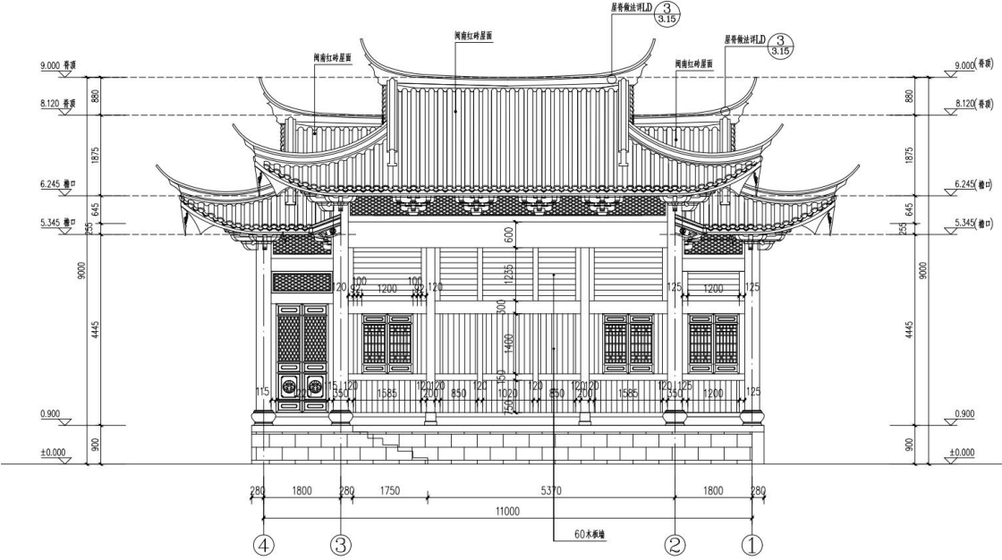
图 3-10 戏台背立面图
