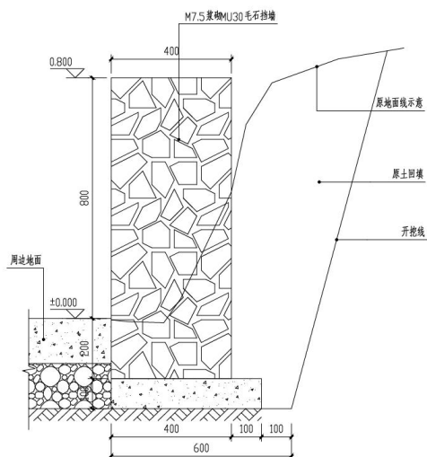
图 3-50 0.8m 高挡墙大样图
