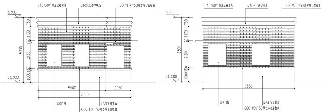
图 3-15 水泵房一立面图 C、D
