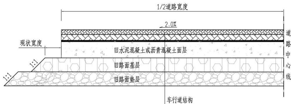
图 3-68 路面改造结构形式一（适用于旧路完好段直接加铺沥青）
